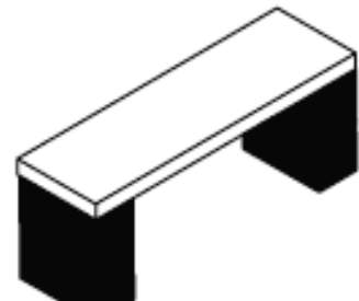
..... CONSOLE TABLE cm. 170 x 56 x h.74 67" x 22" x h.29"
