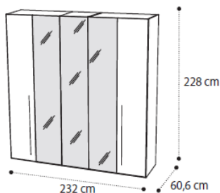
Armadio batt. 5 ante, specchio 5 door glass doors wardrobe Шкаф 5-ти дв. с зеркалами
