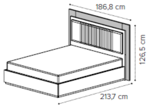
Letto SOFT QS 154 Bed SOFT QS 154 Кровать SOFT QS 154
