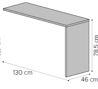
Toilette Vanity extension Стол туалетный
