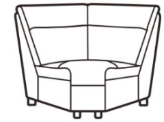
CORNER UNIT H 102cm W 174cm D 100cm SH 49cm SW 31/99 cm SD 52cm Square Corner 124cm x 124cm
