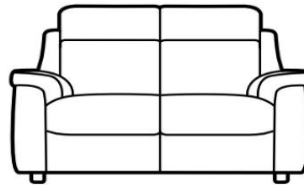
TWO SEATER SOFA H 102cm W 146cm D 100cm SH 49cm SW 98cm SD 52cm AH 63cm
