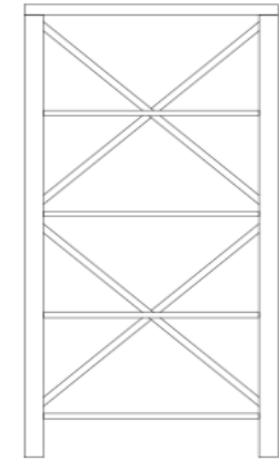
BOOKCASE H 1750 W: 800 D: 375
